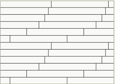
Regular laying (secuencia: 1-3-4, 3-6-7, 3-9-12 cm.) Colocación regular
